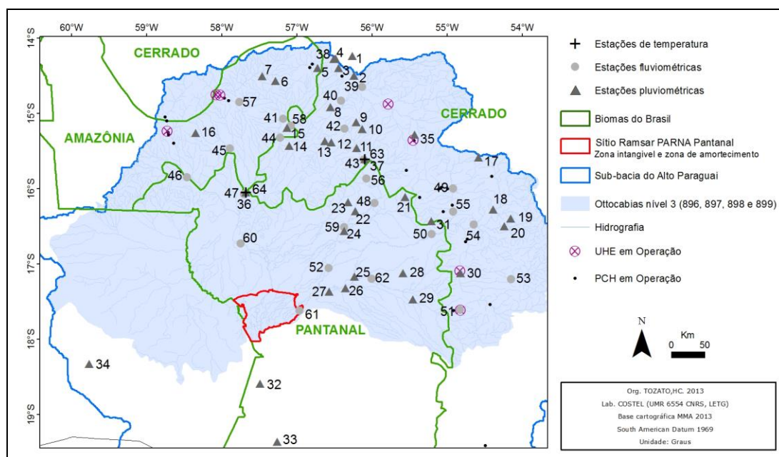
Figura 3. Localização das estações de pluvimetria, cotas fluviométricas e de temperatura na sub-bacia do Alto Paraguai, no bioma Pantanal. 1-38=estações pluviométricas; 39-62=estações fluviométricas; 63-64=estações de temperatura. 1=Diamantino (1456005), 2=Rosário Oeste (1456008), 3=Diamantino (83309), 4=Nortelândia (1456003), 5=Quebo (1456004), 6=Tangara da Serra (1457001), 7=Tapirapuã (1457000), 8=Parecis (1456009), 9=Acorizal (1556005), 10=Nossa Sra da Guia (1556000), 11=Nossa Sra do Livramento (1556001), 12=Seco (1556006), 13=Cuiabá (1556002), 14=Barra do Bugres (1557001), 15=Porto Estrela (1557000), 16=Alto Jauru (1558004), 17=Jacara (1554006), 18=Rondonópolis (1654000), 19=Santa Terezinha (1654001), 20=Santa Escolástica (1654004), 21=Barão de Melgaço (1655002), 22=Porto Cercado (1656001), 23=Poconé (1656002), 24=São João (1656004), 25=São José do Piquiri (1756001), 26=Ilha Camargo (1756000), 27=Porto do Alegre (1756003), 28=São Jerônimo (1725003), 29=União (1755001), 30=Itiquira (1754000), 31=Itaipu (1655003), 32=Porto Suarez (1683), 33=Porto Esperança (1957006), 34=Robore (1728), 35=Chapada dos Guimarães (1555001), 36=Cáceres (83405), 37=Cuiabá (83361), 38=Arenópolis (1456001); 39=Quebo (66160000), 40=Rosário Oeste (66250001), 41=Barra do Bugres (66010000), 42=Acorizal (66255000), 43=Cuiabá (66260001), 44=Porto Estrela (66015000), 45=Estrada MT-125 (66065000), 46=Porto Esperidião (66072000), 47=Cáceres (66070004), 48=Barão de Melgaço (66280000), 49=São Pedro da Cipa (66380000), 50=Acima Córrego Grande (66460000), 51=Estrada BR-163 (66490000), 52=Ilha Camargo (66370000), 53=Itiquira (66520000), 54=Rondonópolis (66450001), 55=São Lourenço de Fatima (66400000), 56=Santo Antônio do Leverger (66270000), 57=Tapirapuã (66050000), 58=Jacara (66080000), 59=Porto Cercado (66340000), 60=Descalvados (66090000), 61=Porto do Alegre (66750000), 62=São Jerônimo (66600000); 63=Cuiabá (83361), 64=Cáceres (83405).
