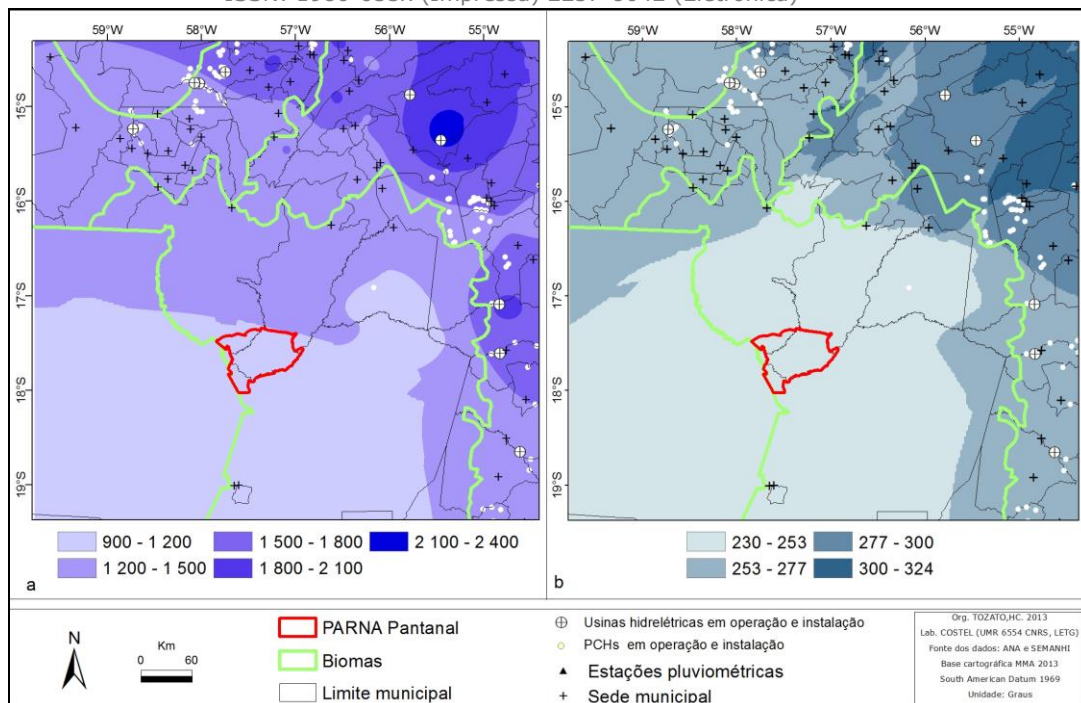
Figura 2. Chuva acumulada na sub-bacia do Alto Paraguai no período de 1971 a 2011. a=pluviometria média anual (mm), b=desvio padrão da pluviometria média anual (mm).
