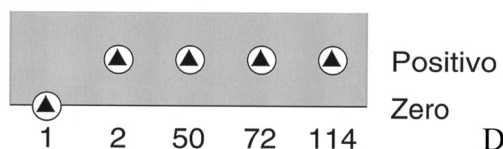
Lagoa: Sedimento removido
