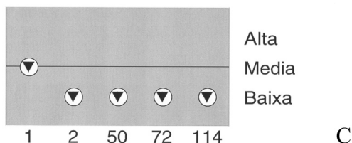
Lagoa: Velocidade da água
