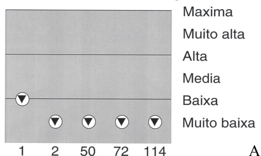
Lagoa: Quantidade de baixios, pontais e ilhas
