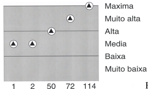
Figura 10 - História de valores dos parâmetros físico-químicos da lagoa: (A) Concentração de nitrogênio; (B) Profundidade; (C) Quantidade de pontais, baixios e ilhas; (D) Sedimento removido; (E) Velocidade da água; (F) Incidência de vento. Os números abaixo dos diagramas se referem ao número de cada estado produzido a partir da simulação. Como existem ambiguidades, estes não estão ordenados consecutivamente.
