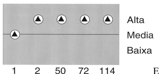
Figura 10 - História de valores dos parâmetros físico-químicos da lagoa: (A) Concentração de nitrogênio; (B) Profundidade; (C) Quantidade de pontais, baixios e ilhas; (D) Sedimento removido; (E) Velocidade da água; (F) Incidência de vento. Os números abaixo dos diagramas se referem ao número de cada estado produzido a partir da simulação. Como existem ambiguidades, estes não estão ordenados consecutivamente.
