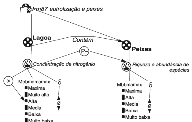
Figura 6 - Fragmento de modelo representando os efeitos negativos da quantidade de nitrogênio na riqueza de espécies de peixes. Lê-se: se lagoa contém Peixes e a Concentração de nitrogênio for maior do que "Alta", a Concentração de nitrogênio afeta negativamente a Riqueza e abundância de espécies de Peixes.
